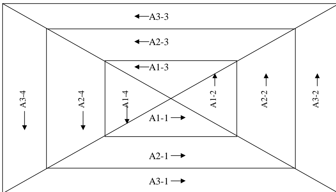
图 6.1.1-3 (a) 方形拼花由里向外逆时针编号排版图
