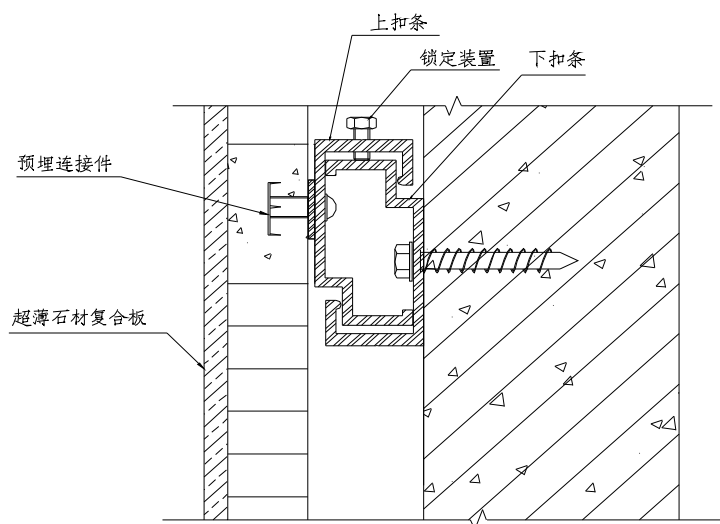
图 7.7.3-3 扣条干挂式
