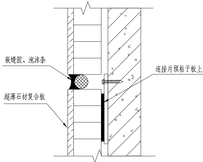
图 7.7.3-2 有连接片粘结式
