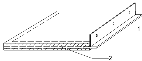
图 7.11.4-2 通挂式示意图
