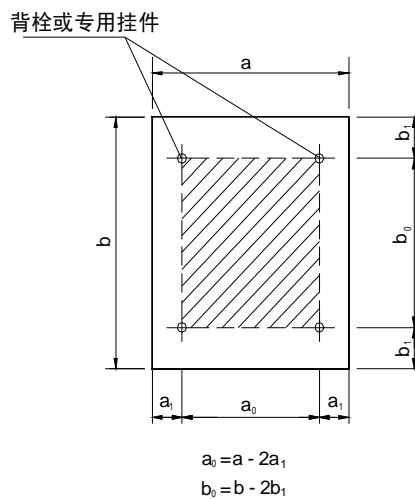
图 4.4.5 背栓及专用挂件连接石板的计算边长
