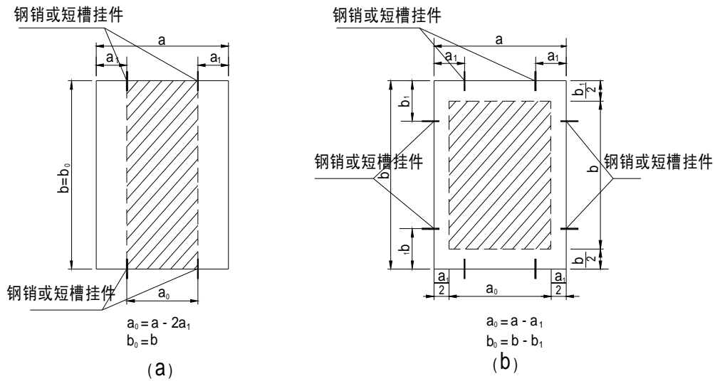
图 4.4.4-1 钢销及短槽挂`连接石板的计算边长
