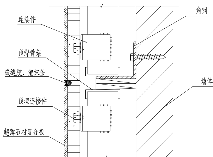
图 7.7.3-4 龙骨固定式
