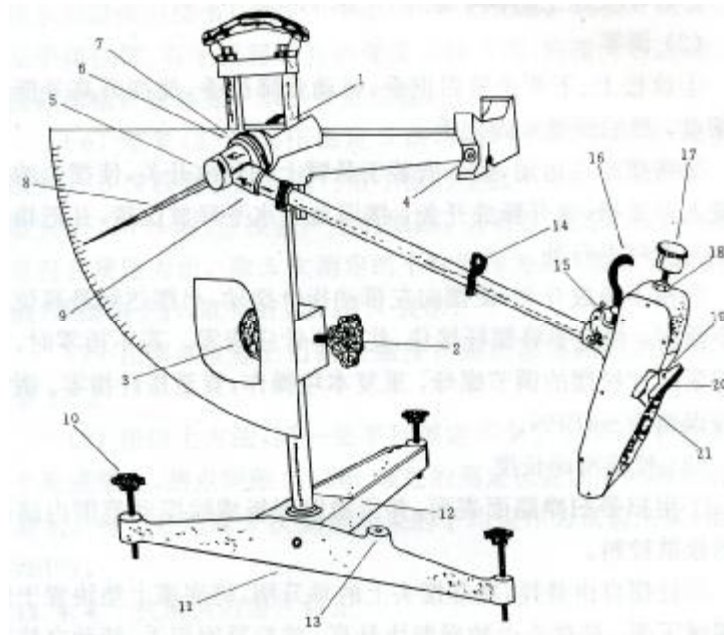
图 E.2.1 摆式仪结构图
