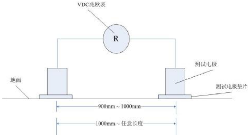
图 A.1.5—1 表面两点间电阻测试
