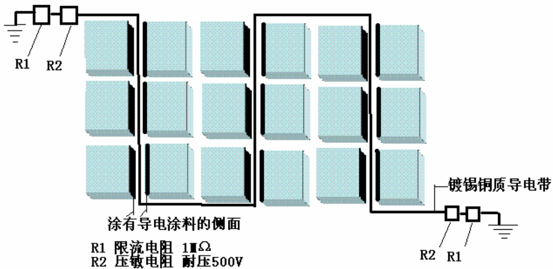
图 7.8.4 预制防静电水磨石板铺装及接地示意图
