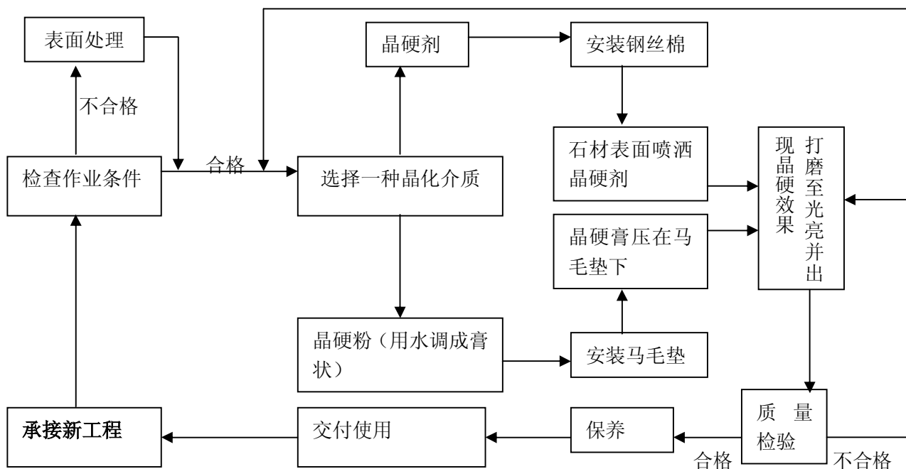
图 8.2.3 晶化处理工艺流程图
