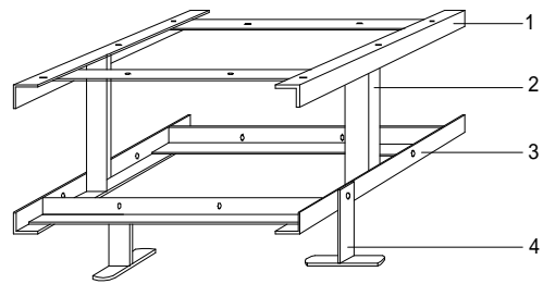
图 7.11.4-1 钢骨架示意图
