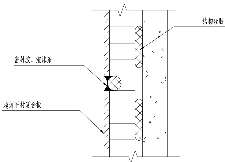
图 7.7.3-1 粘贴式
