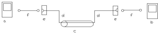
图 4.4.3-1 光纤链路测试连接图
