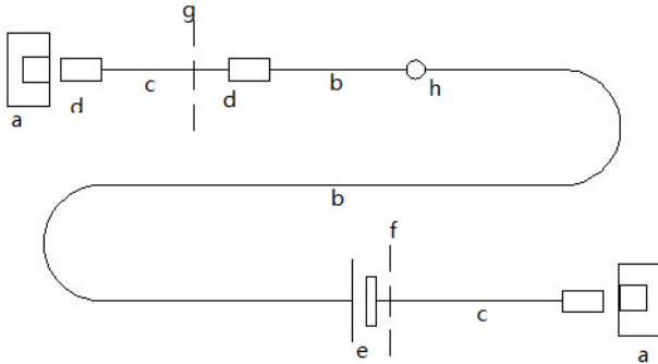
图 4.4.2-1 永久链路测试连接图
