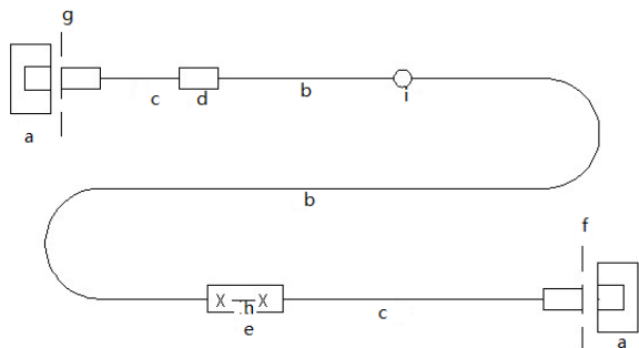
图 4.4.2-2 信道测试连接图
